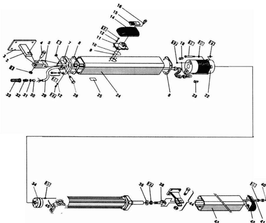
Vista explosa
