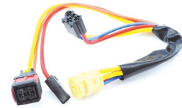
Ref.RS377 CONTACTOR ARRANQUE PEUGEOT 406 (BI578)
