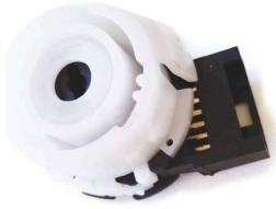
Ref.RS307 CONTACTOR ARRANQUE VW/AUDI VARIOS (1K0905865A)
